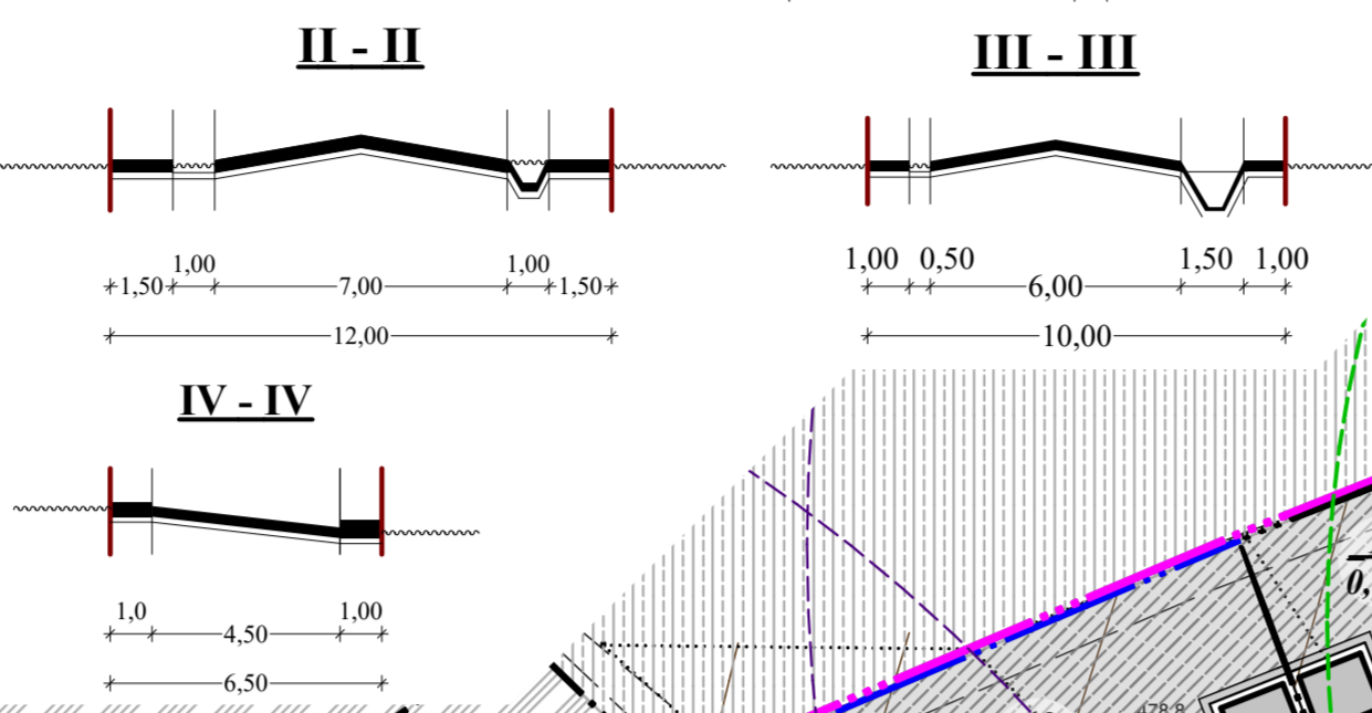
ПОПЕРЕЧНІ ПРОФІЛІ ВУЛИЦЬ ТА ПРОЇЗДІВ М 1:200
