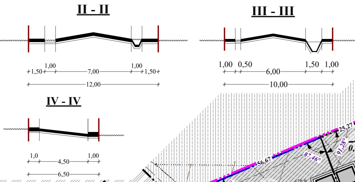
ПОПЕРЕЧНІ ПРОФІЛІ ВУЛИЦЬ ТА ПРОЇЗДІВ М 1:200
